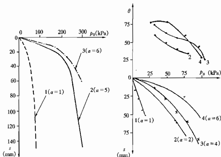
图 5 现场载荷试验 p-s 曲线
